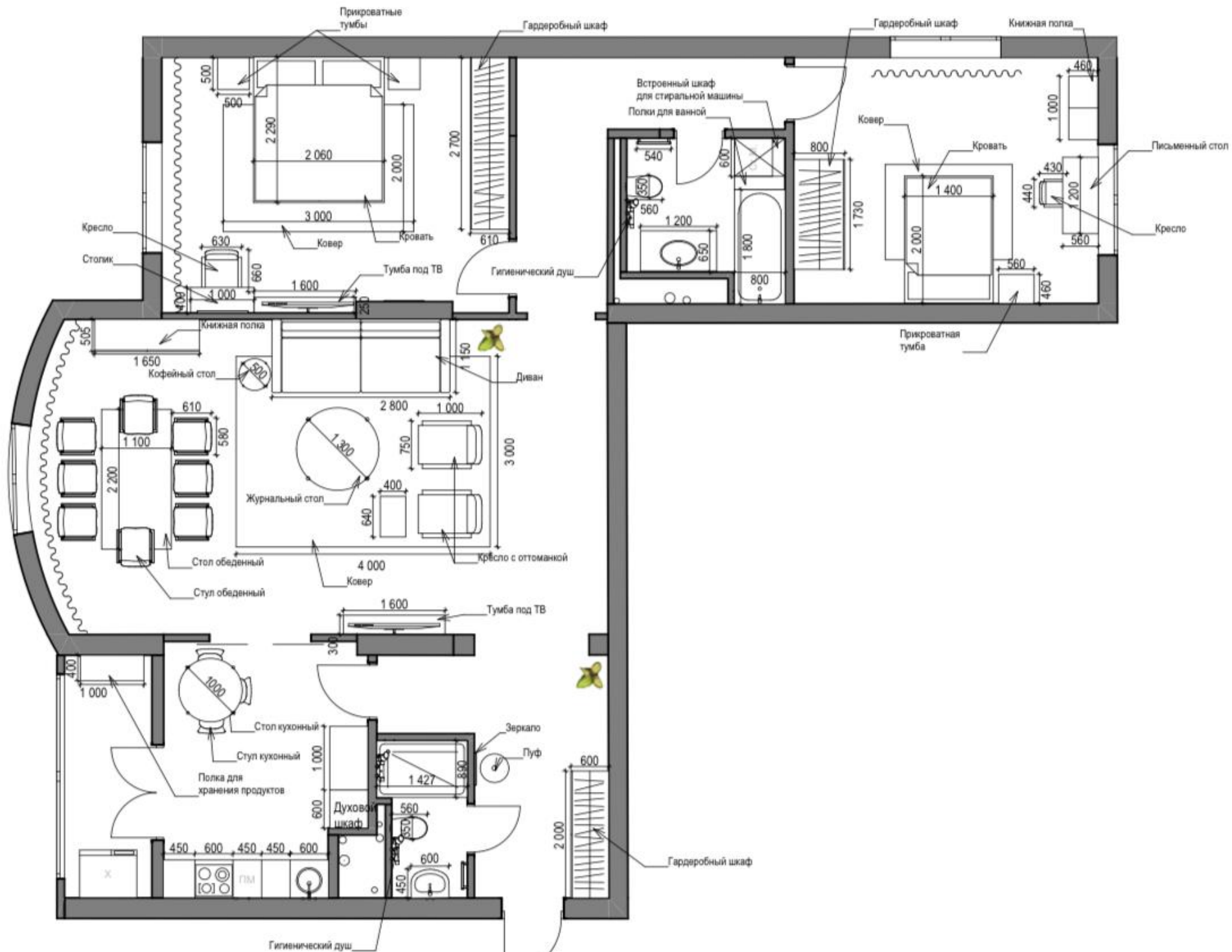
План расстановки мебели с размерами
